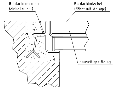
Typ 8: Baldachinabschluss oben eben • nur in trockenen Bereichen • mit Wanne für bauseitigen Belag zur optischen Anpassung an den vorhandenen Boden
