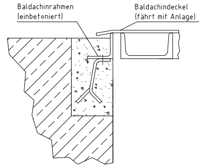
Typ 5: Baldachinabschluss oben aufragend • Wassereintritt konstruktiv reduziert • für Innen - und Außenbereiche
