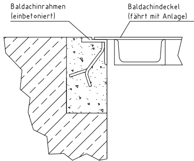
Typ 3: Baldachinabschluss oben eben • vorwiegend innerhalb von Gebäuden • nicht für Nassbereiche geeignet
