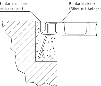
Typ 7: Baldachinabschluss oben eben • mit umlaufender Wasserablauffrinne zur Aufnahme von Oberflächenwasser
