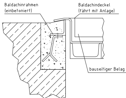
Typ 5W: Baldachinabschluss oben aufragend • mit Wanne für bauseitigen Belag zur optischen Anpassung an den vorhandenen Boden
