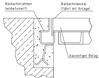
Typ 8E: Baldachinabschluss oben eben • mit umlaufender Wasserablauffrinne zur Aufnahme von Oberflächenwasser • mit Wanne für bauseitigen Belag zur optischen Anpassung an den vorhandenen Boden
